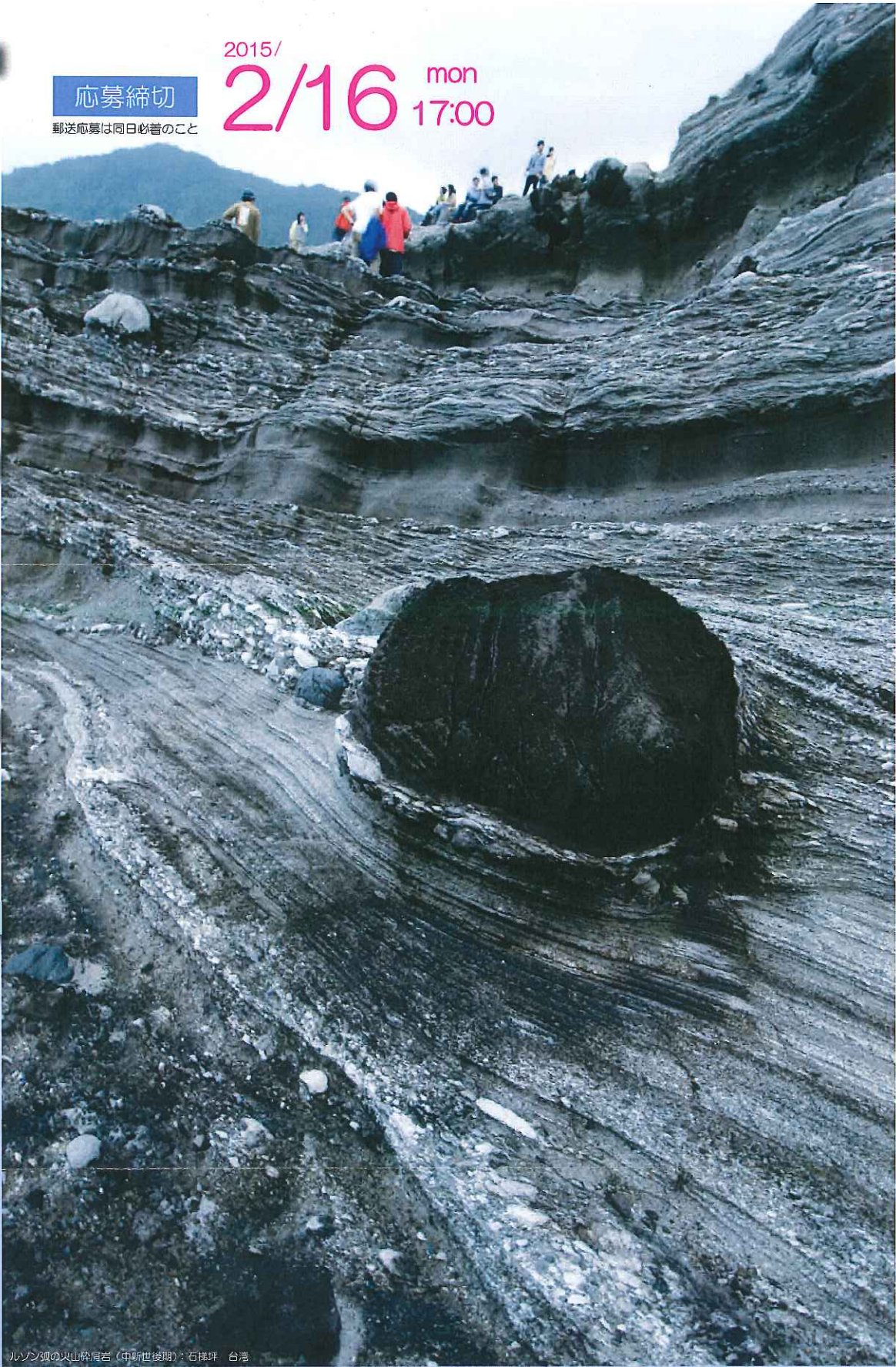
ルソン領の火山砕屑岩(中新世後期):石碇坪 台湾
